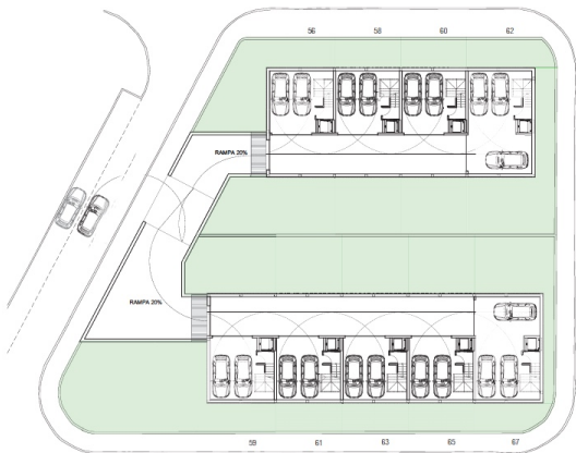
PLANTA SOTERRANI ↻
