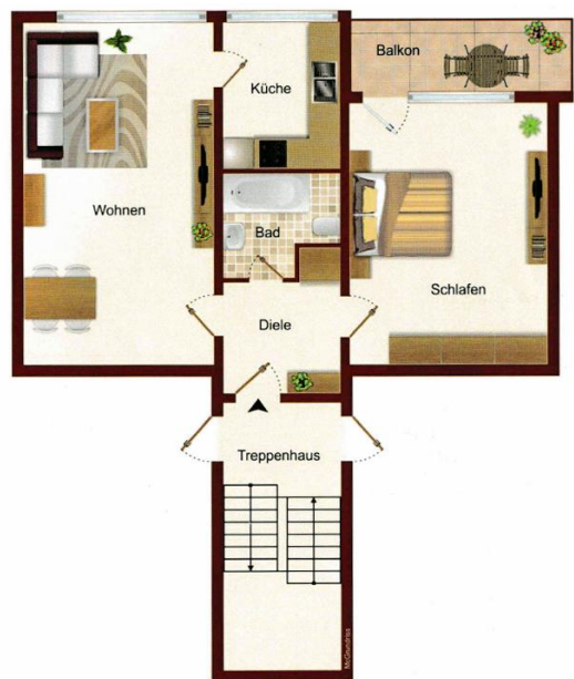
Grundriss
